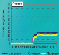
Динамика дефектов
